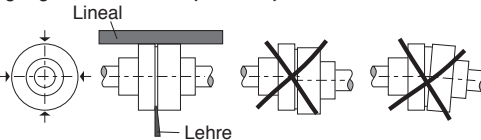
Abb. 6A Kupplungsausrichtung.
