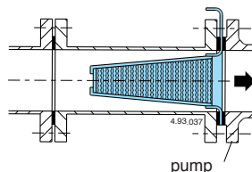
Bild 5 Tillfällig konisk filter i sugledningen.
